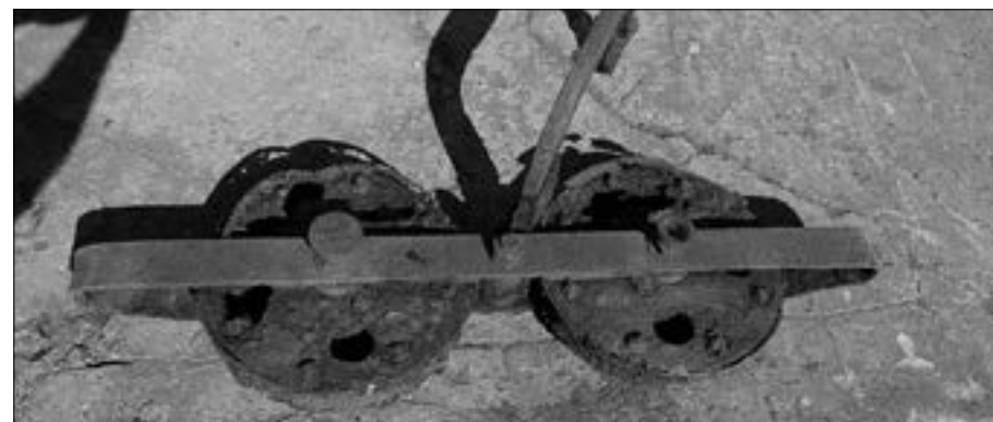
Nalezený původní běhoun nákladní visuté dvoulanové dráhy oběžného systému, která měla tři izolované úseky, denní přepravní kapacitu 100 tun, šířkou délku 4 000 m, překonávající převýšení 500 m.
